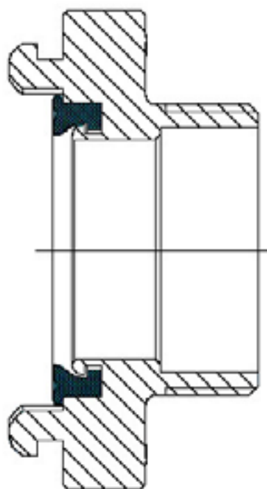
RACCORD MÂLE
